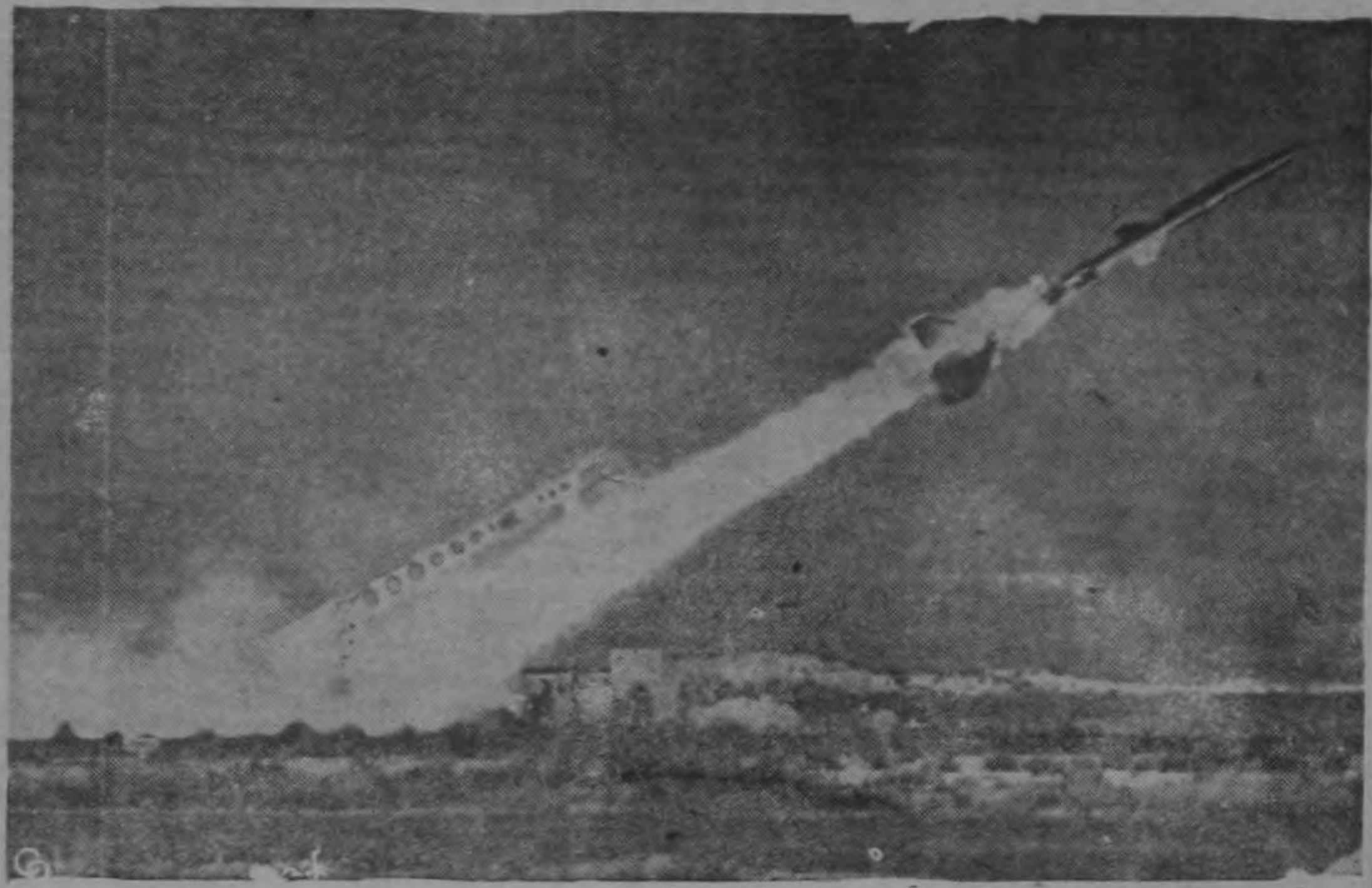
Un "GAPA" supersónico Boeing gana velocidad después de ser lanzado en un experimento en Alamogordo, Nuevo México. Esta foto fué dada a la publicidad con aprobación del Departamento de Defensa de Washington después de anunciarse que hace más de cinco años que los Estados Unidos están haciendo experimentos con proyectiles guiados anti-aéreos que desarrollan 2.400 kilómetros por hora.—(INP).
